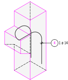
Stabform: "Konsolenisen"
