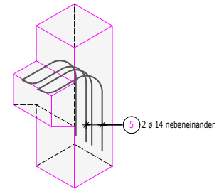
"Konsolenisen"
