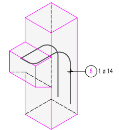
"Konsolenisen"
