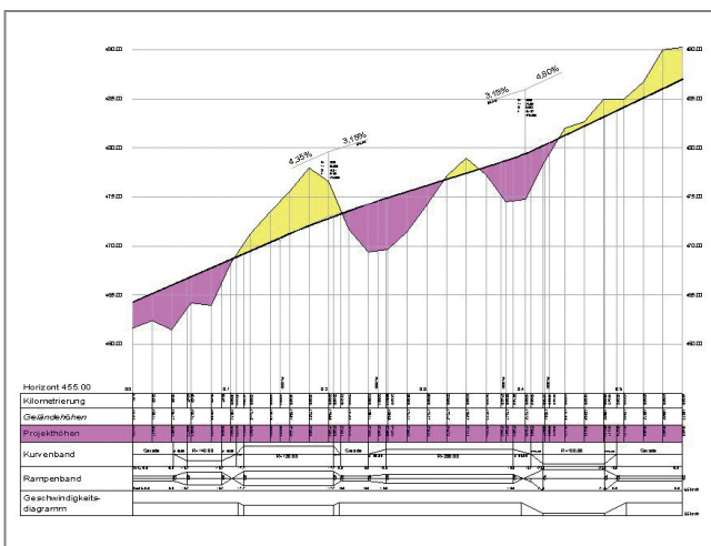
Lageplan, Höhenplan und Querprofile werden aus dem 3D-Modell abgeleitet. (Höhenplan Zufahrtsstrasse Payerne, Département des Infrastructures, Lausanne, CH)
