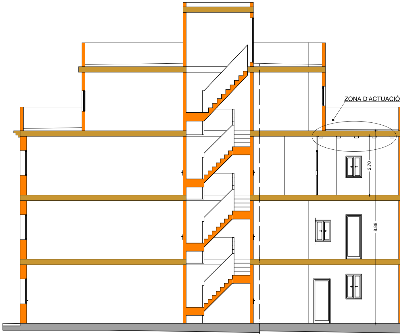
Secció L2 - L2
