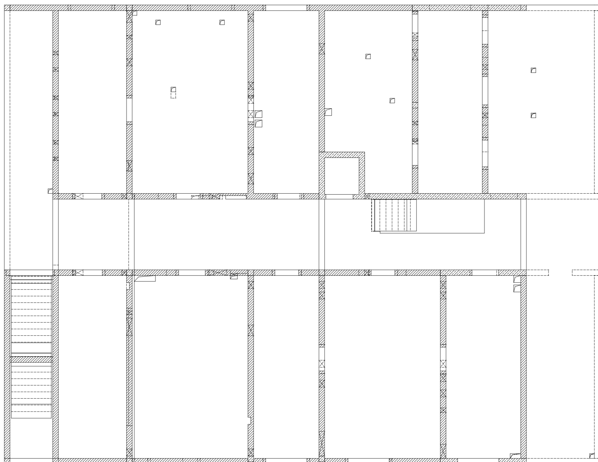
DECKENUNTERSICHT 1-1
