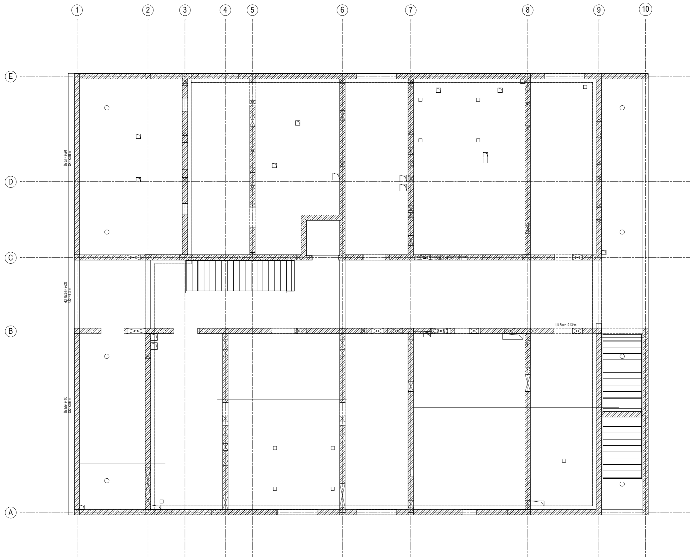
DECKENUNTERSICHT 1-1
