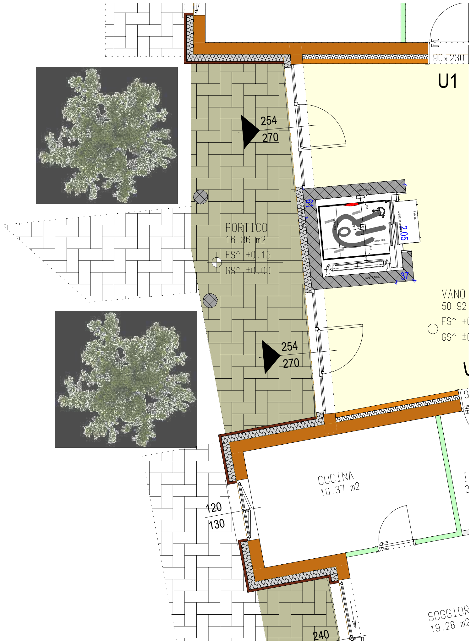
PLANIMETRIA PROGETTO - Scala 1 : 0.50
